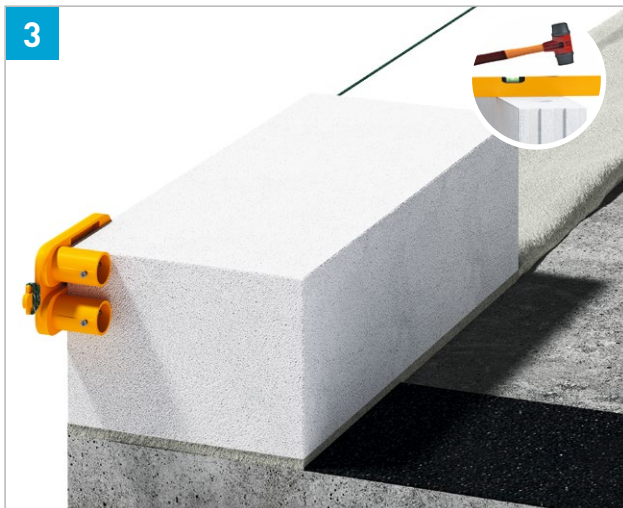
Setzen und Ausrichten der Ausgleichsschicht in Normalmauermörtel M10 nach DIN 20000-412 (vormals MG III) (Dicke der Mörtelfuge von 1 bis 3 cm). Anlegen des Mauerwerks immer nach Robaumaß
