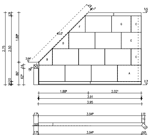
Wand Nummer 131 mit Giebelschräge und Gehrungsschnitt
