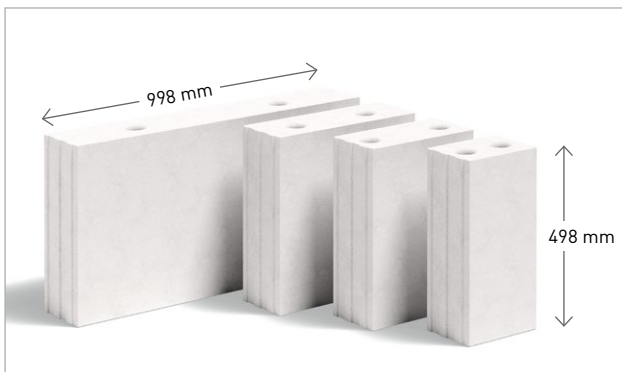
Silka XL-Regel- und Ergänzungselemente, Höhe 498 mm
