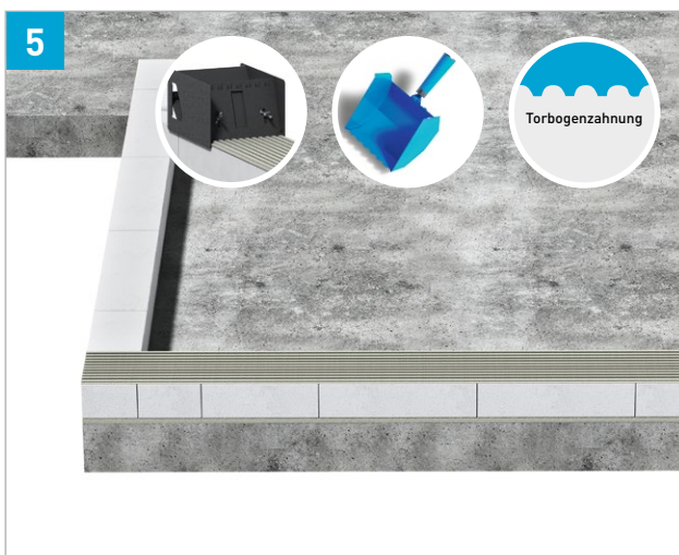
Silka FIX S202 (Silka Secure Dünnbettmörtel) auftragen
