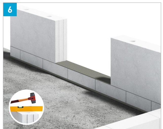
Ecksteine setzen und ausrichten
