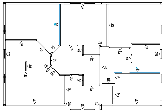
Planungsbeispiel: Grundriss mit Wand-Nummerierung und Blickrichtung
