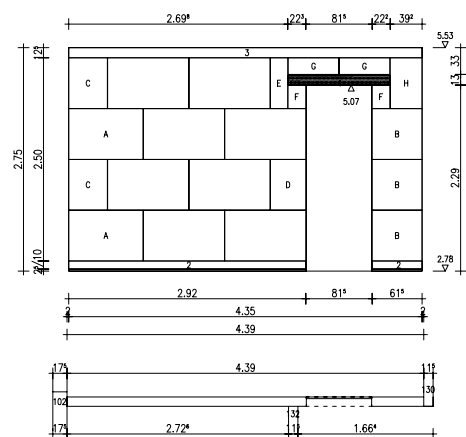
Wand Nummer 112 mit Türöffnung und Sturz
