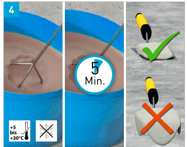
Silka FIX S202 (Silka Secure Dünnbettmörtel) anmischen (Reifezeit und Konsistenz beachten)
