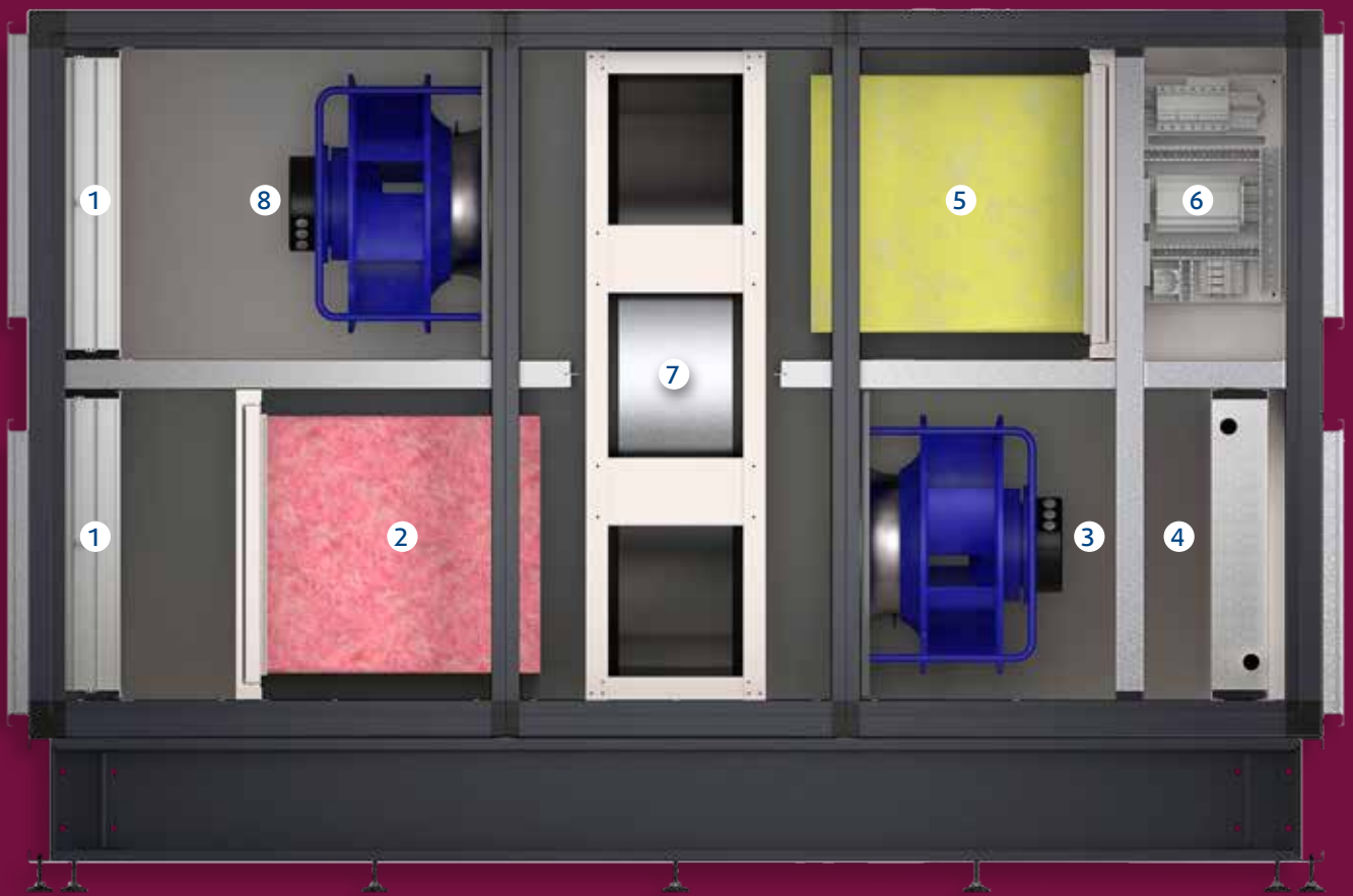
Geniox-Zeichnung
