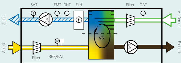
SAVE VSR 500 *
