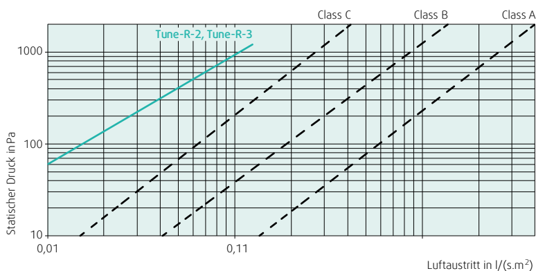
Diagramm 2: Klassifizierung der Leckage nach EN 1751
