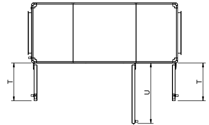
Topvex SC06
