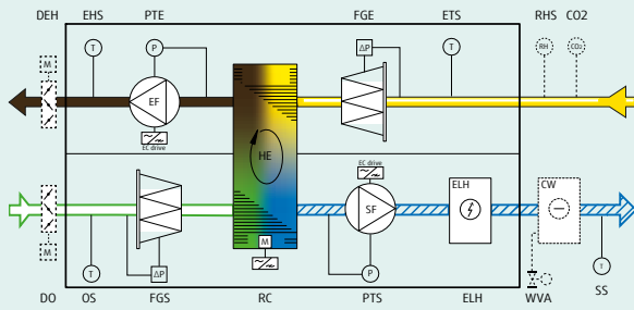
Topvex SR03-11EL-R-CAV
