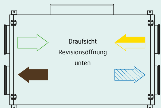
Rechte Ausführung
