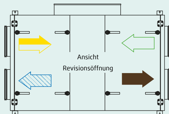
Rechte Ausführung
