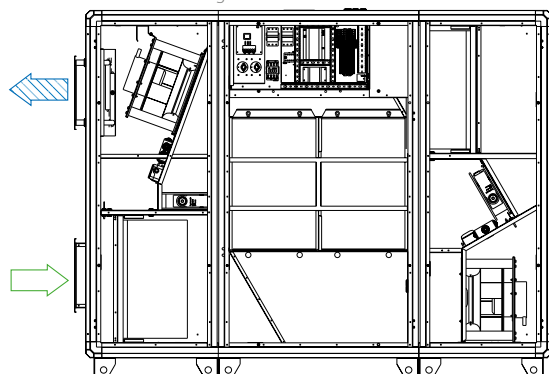
linke Ausführung
