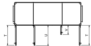
Topvex SC08
