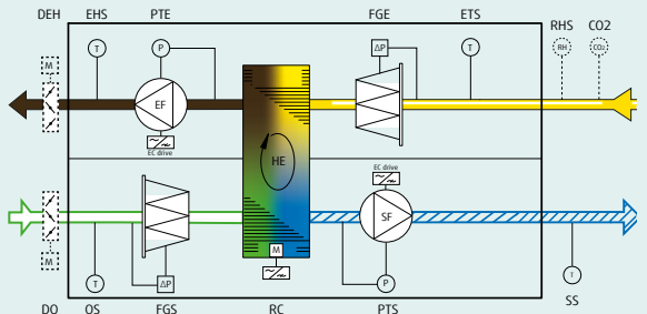
Topvex SR03-11R-CAV
