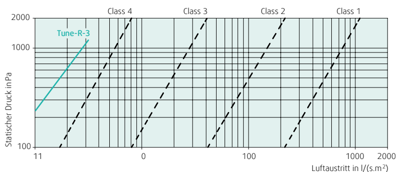
Diagramm 1: Klassifizierung der Leckage von geschlossenen Klappen gemäß EN 1751
