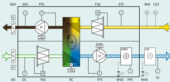
Topvex SR03-11HW-R-CAV
