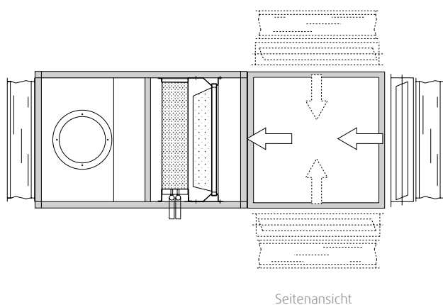
Seitenansicht
