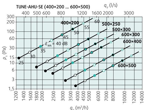
Diagramm 1: Druckverlust und A-bewerteter Gesamtschallpegel in Abhängigkeit vom Luftvolumenstrom; durch offene Klappe
