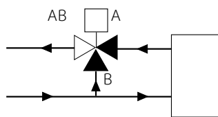
3-Wege-Ventil
