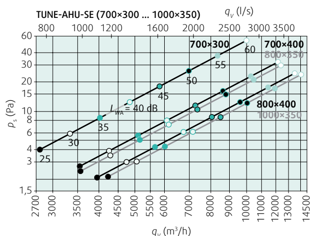
Diagramm 2: Druckverlust und A-bewerteter Gesamtschallpegel in Abhängigkeit vom Luftvolumenstrom; durch offene Klappe
