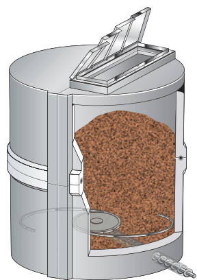
Mall-Hackschnitzelspeicher z.B. ThermoPal 60000
