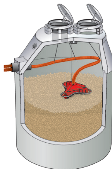
Mall-Pelletspeicher Maulwurf 3000 - E3
