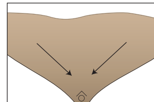
Herkömmlich: Pellets werden zur Entnahme bewegt, Entmischung von Pellets und Feinanteil
