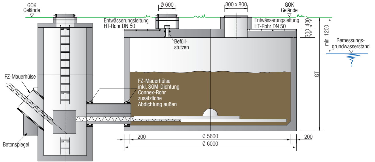
Mall-Revisionschacht rund
