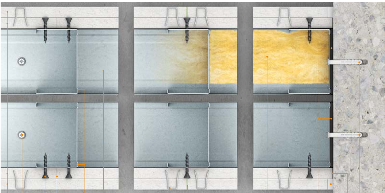
1 12,5 mm fermacell® Firepanel A1
