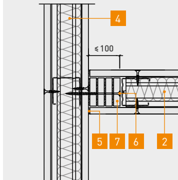
1 S 21 fermacell™ Montagewand
