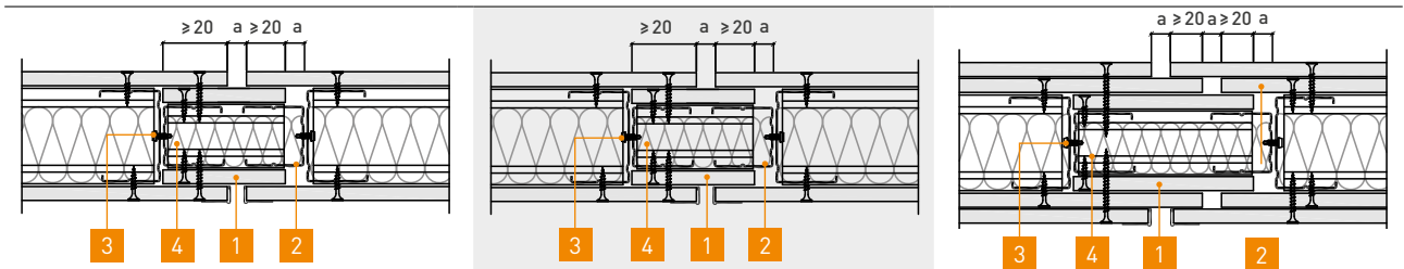
1 S 15 fermacell™ Montagewand
