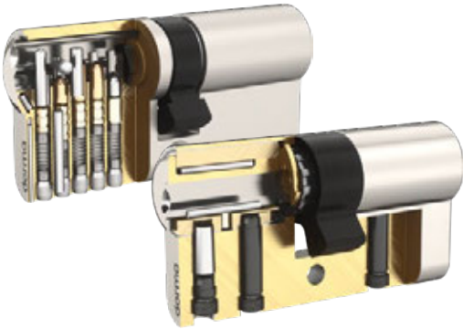
Schließzylinder mit erhöhtem Bohrschutz (BS)
