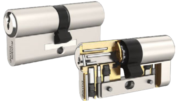
Zackenschlüsselsystem mit Lamellenausführung und Wendeschlüsselsystem mit erhöhtem Bohr- und Ziehschutz (BZ-LAM)
